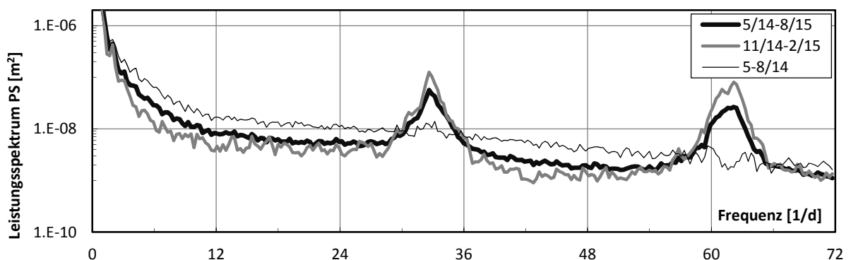
Abb. 11 Leistungsspektrum des Zürichseepegels am Zürichhorn mit saisonaler Aufteilung.
