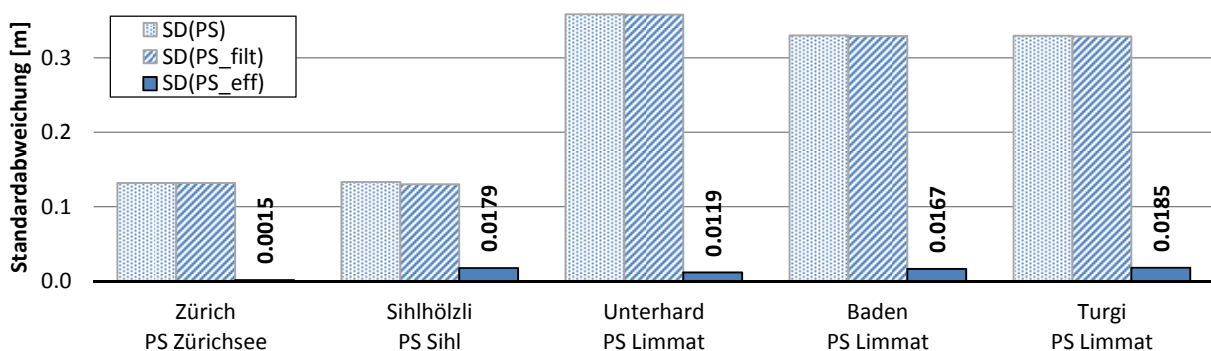
Abb. 7 Vergleich der Standardabweichung der kurz- und langperiodischen Pegelschwankungen entlang der Messstellen flussabwärts der Limmat
