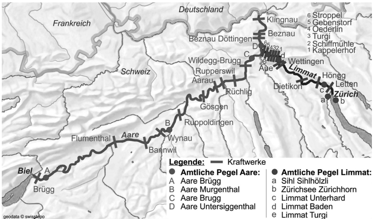
Abb. 1 Übersichtsplan Aare und Limmat mit Zuflüssen, Kraftwerken und Messstellen.
