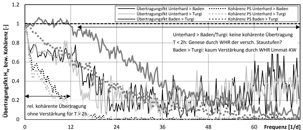
Abb. 10 Übertragungsfkt. und Kohärenz der Pegelschwankungen in Funktion der Frequenz.
