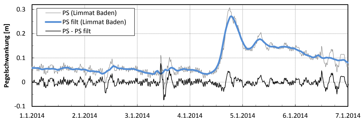
Abb. 2 Pegelschwankungen (PS), Filterung (PS filt) und result. Differenz (PS-PS filt).
