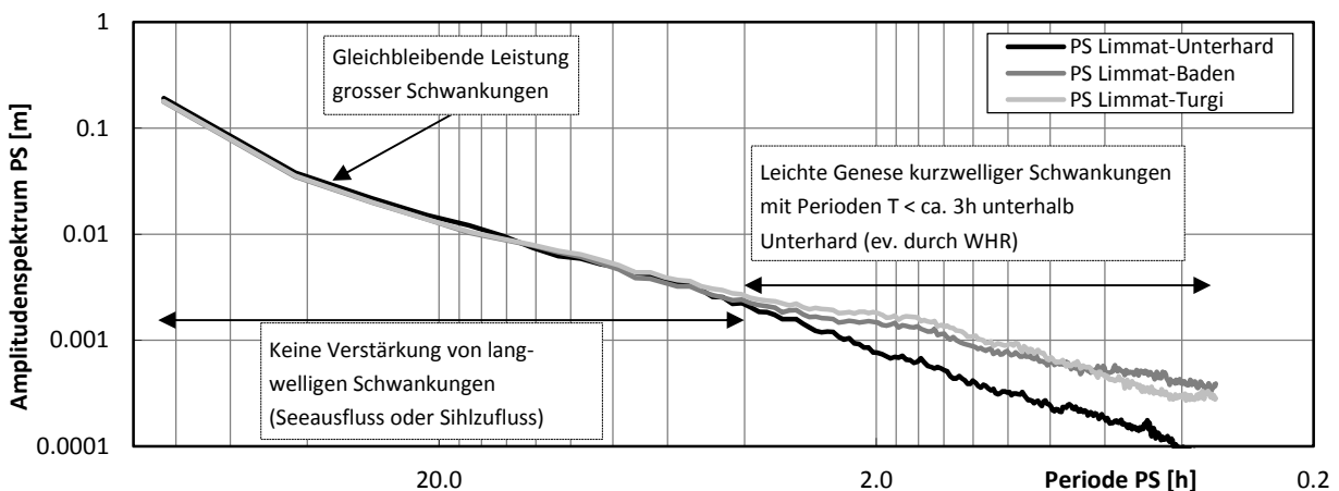
Abb. 9 Amplitudenspektrum Pegelschwankungen in Funktion der Wellenperiode ( 1/f ).
