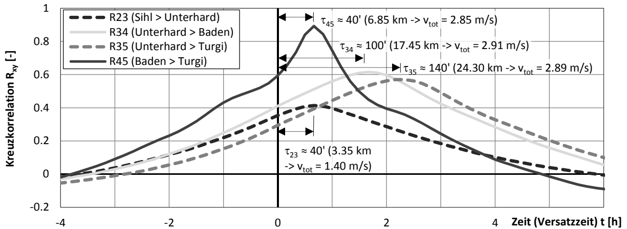
Abb. 8 Kreuzkorrelation und Phasen- d.h. Zeitversatz der Pegelschwankung.
