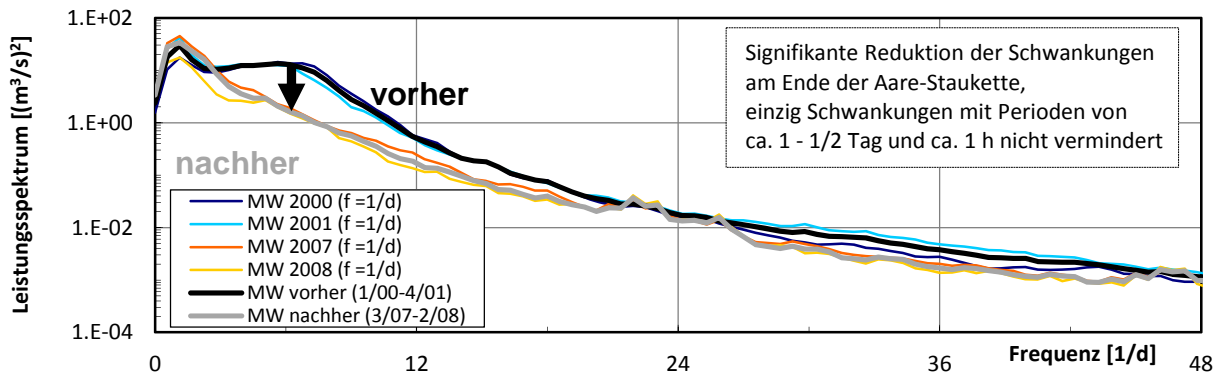
Abb. 5 Leistungsspektren der Q-Schwankungen (Pegel Brugg) vor und nach Massnahmen.
