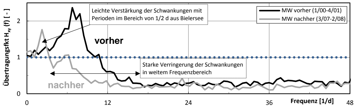
Abb. 6 Übertragungsfunktionen (Brügg-Ägerten -> Brugg) vor bzw. nach Modifikation.
