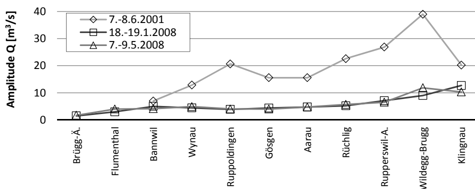
Abb. 4 Mittlere Amplitude der Abflussschwankungen ausgewählter Zeitreihen bei MQ: Vergleich der Situation vor und nach Umsetzung der Massnahmen.
